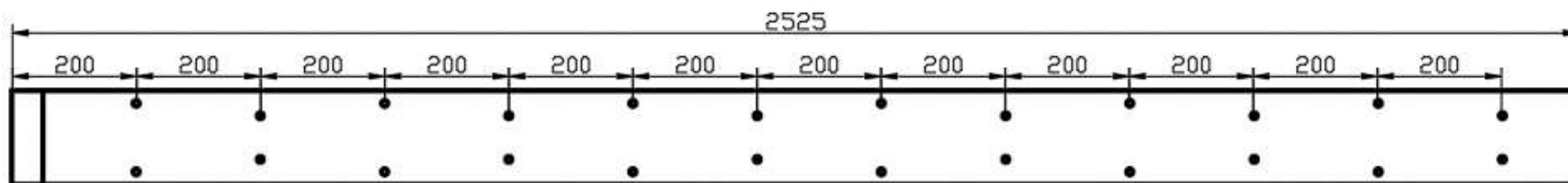
Widok z góry (1:10)
